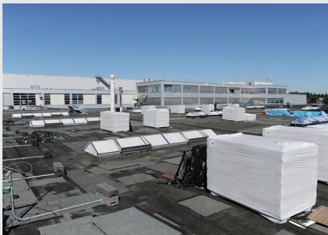
Sanierung einer Lagerhalle mit 7.800 m 2 Dachfläche: Austrocknung des durchfeuchteten Dachschichtenpakets
