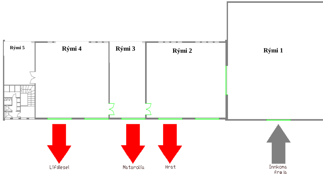
Einföld mynd sem sýnir mögulega uppbyggingu húsnaðisins fyrir verksmiðjuna[2]
