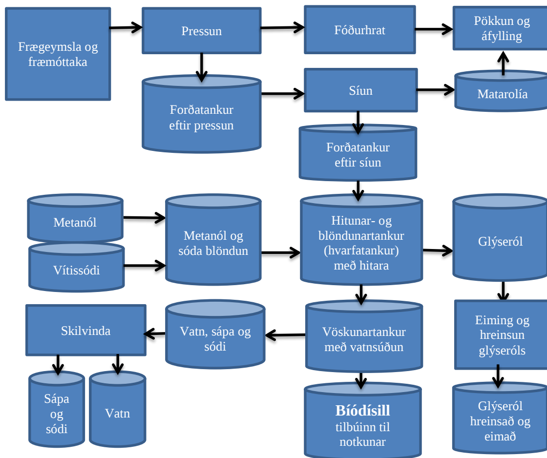
Flæðirit framleiðslunnar[2]
